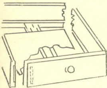
การทำร่องเลื่อนตรงกลางลั่นชัก
