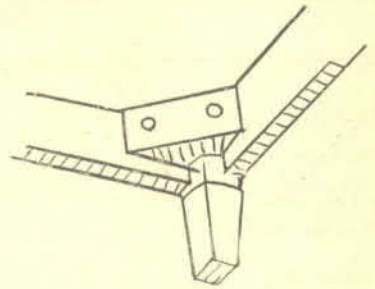
การเข้ามุมใช้ตะปูเกลียว
