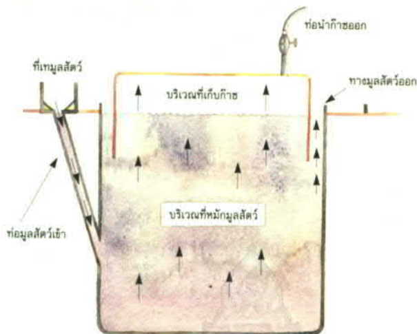
ภาพด้านตัดของบ่อก๊าซชีวภาพ
